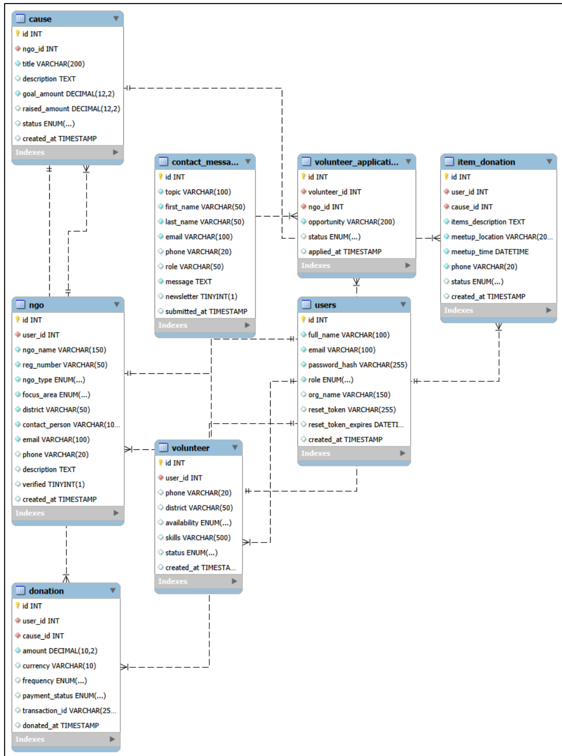
Figure 2: ER Diagram
